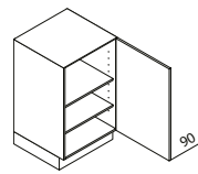
UDD Base unit ↳ 30/40/45/50/60 ↓ 90 ↙ 60/50/39
