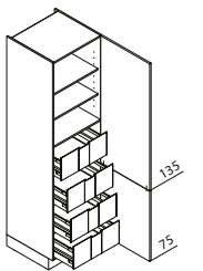
VI Larder unit ↔ 40/45/50/60 ↓ 195/210/225 ↙ 60/50/35
