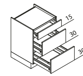
KUAK Hob base unit
