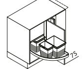
UEPSZ Sink base unit space filler
